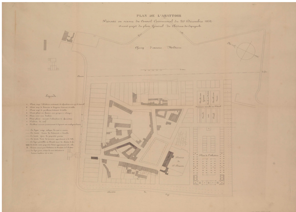
Floor plan of the slaughterhouse and the neighbourhood/Plattegrond van het slachthuis en de buurt
